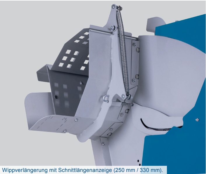
Wippverlängerung mit Schnittlängenanzeige (250 mm / 330 mm).
